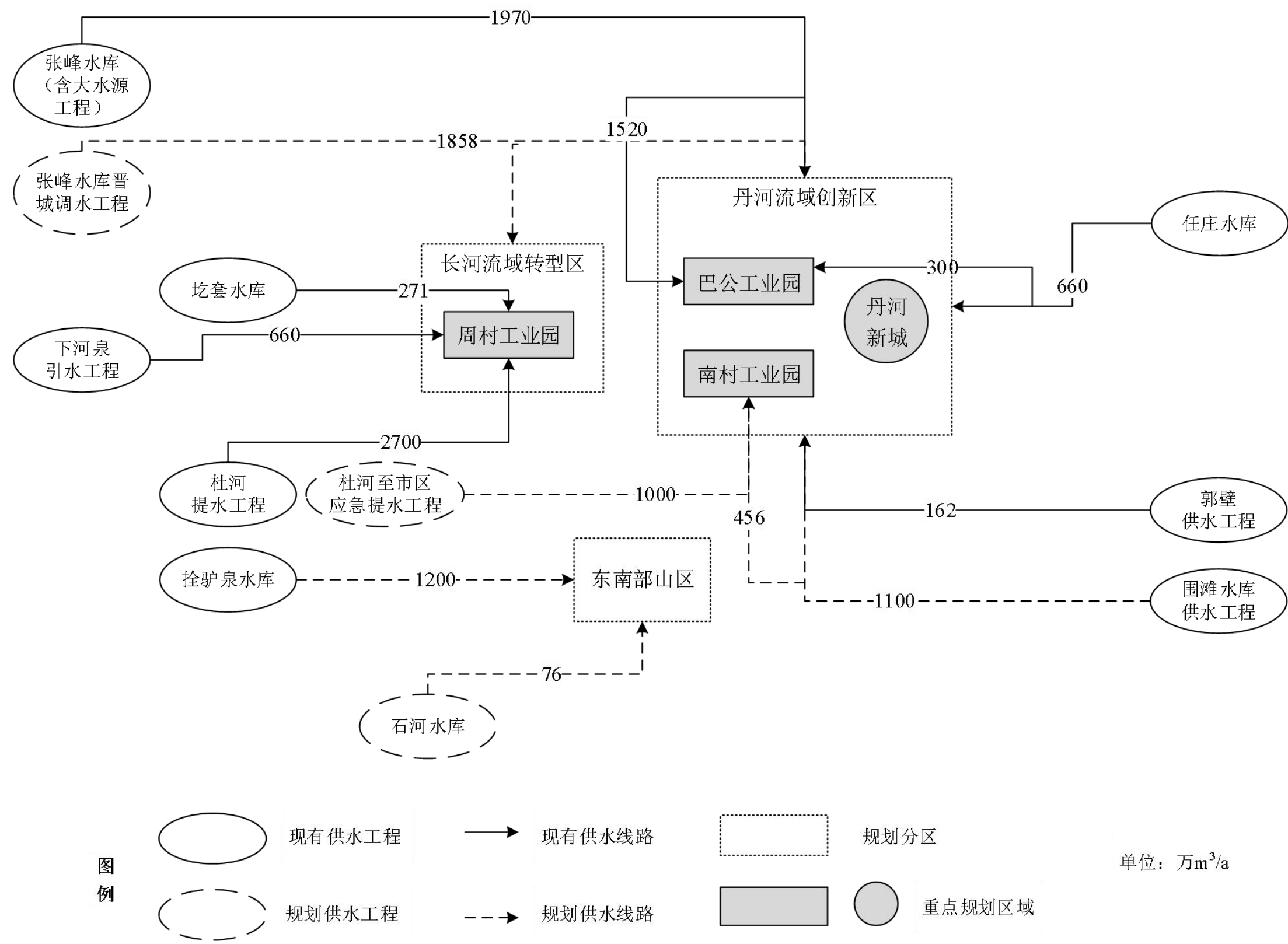
图 7-1 泽州县主要供水工程配置图
