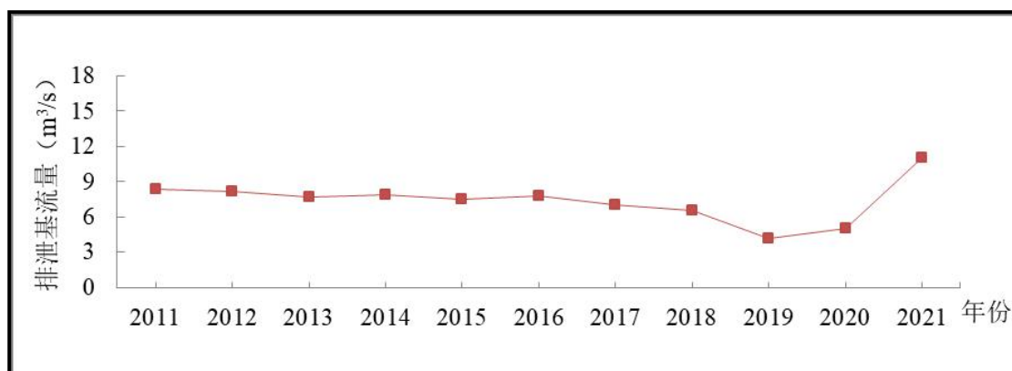
图 3-14 延河泉域 2011-2019 年排泄基流量变化图
