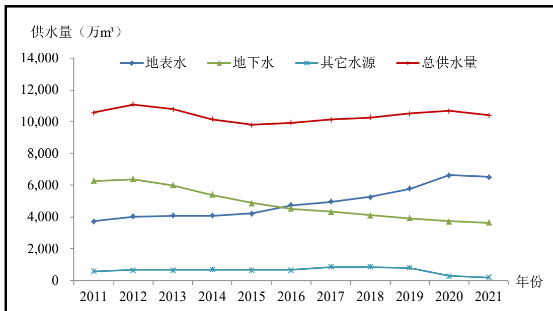
图 3-2 历年供水量变化情况图
