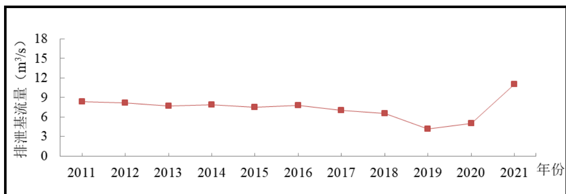
图 3-14 延河泉域 2011-2019 年排泄基流量变化图
